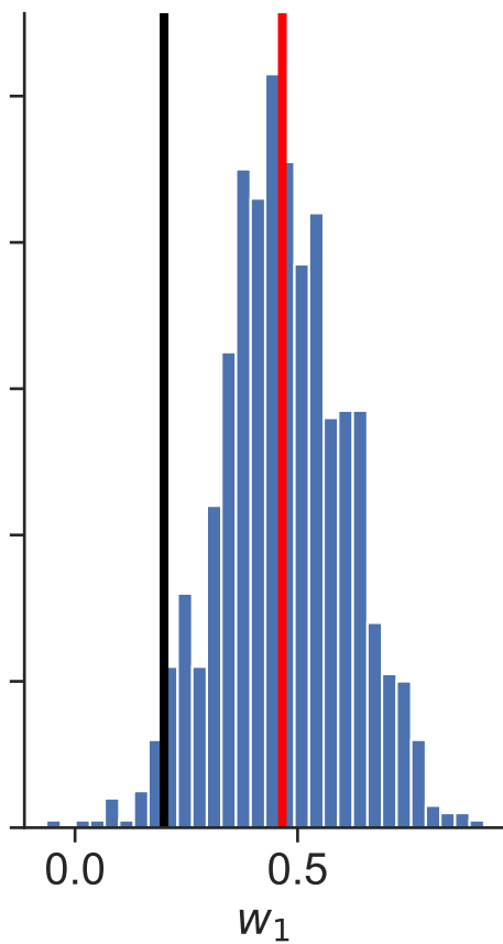
Posterior distributions Dataset 23
